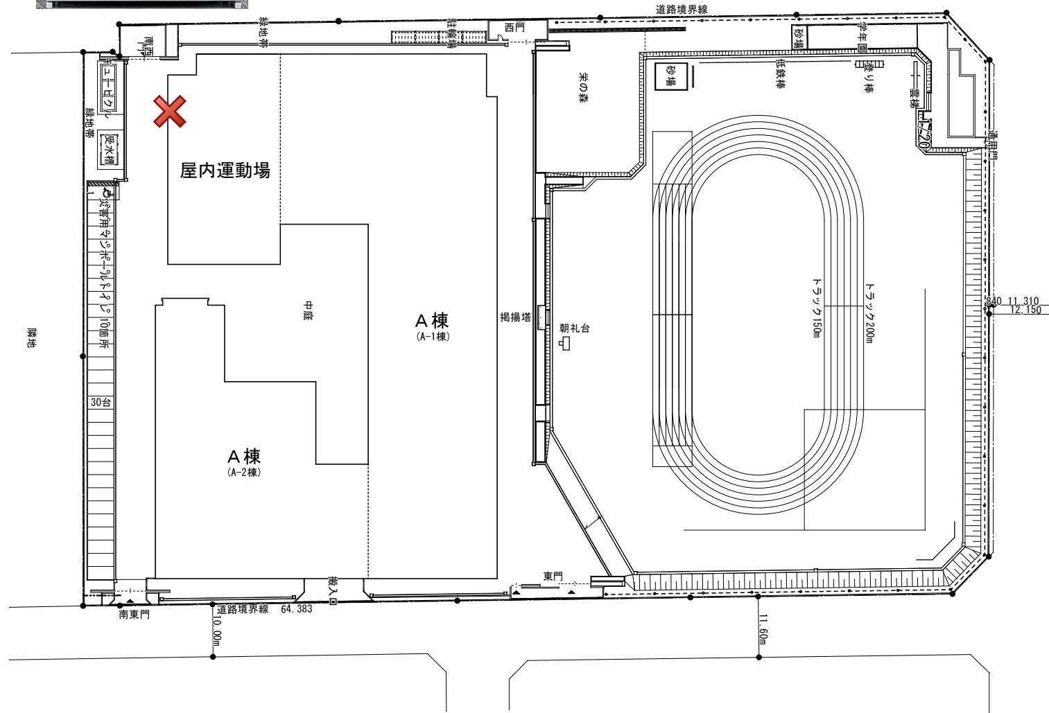
配置図 S=1/1000
